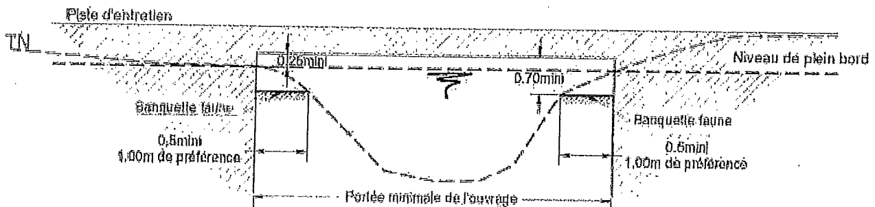
Illustration 1. Schéma de principe du franchissement des Rigoles.
